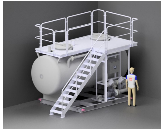
Ensilasjesystem Syrefast
